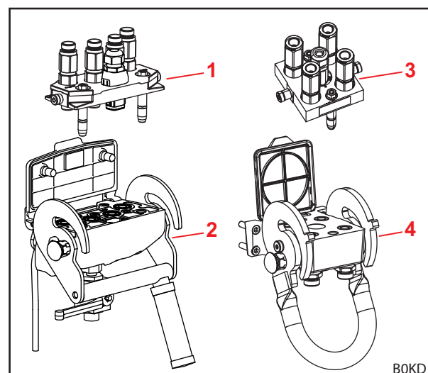
Abb. 23 Aufbau Hydro-Fix und Multikuppler
