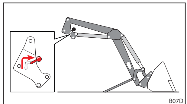
Abb. 46 Frontlader-Verriegelung öffnen
