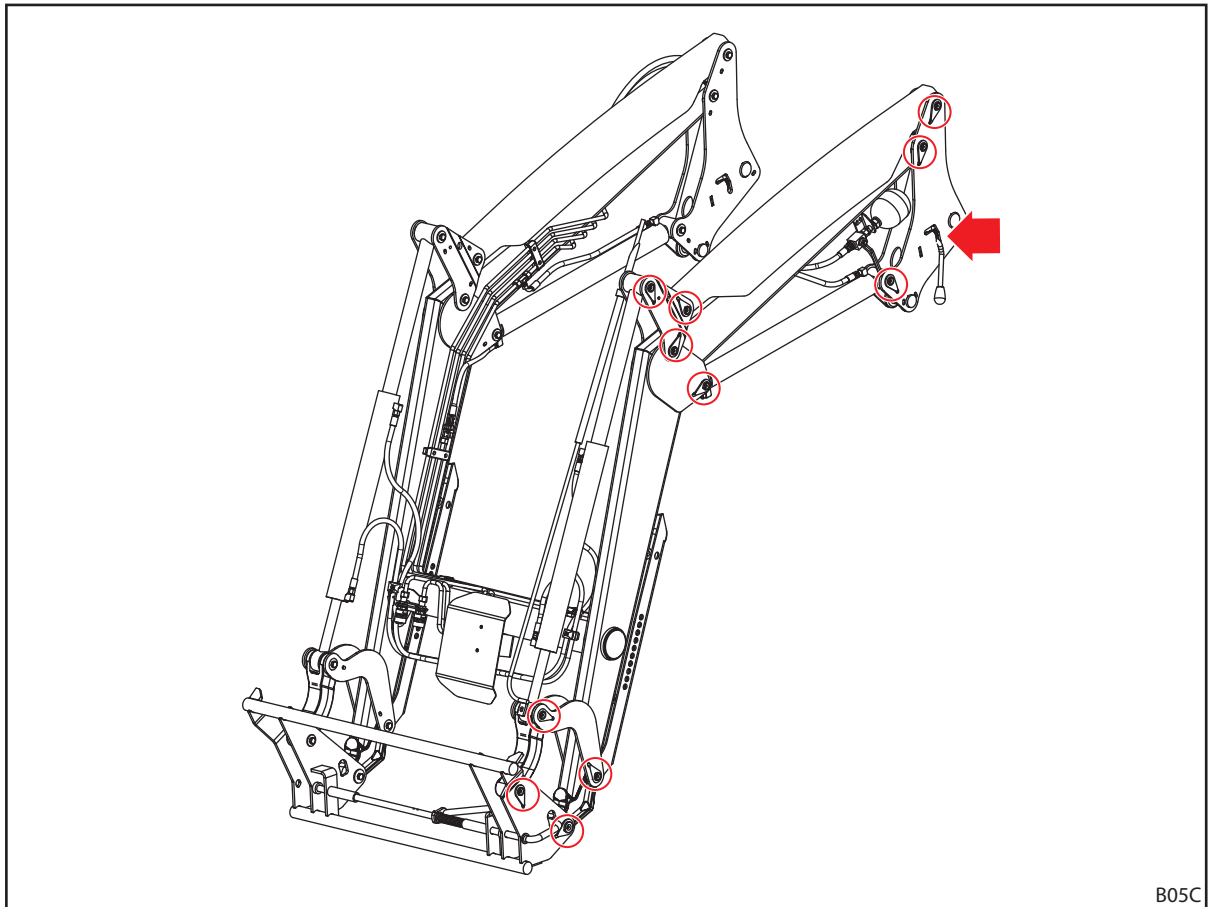
Abb. 110 Schmierstellen P
