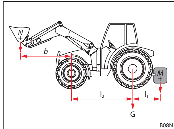
Abb. 45 Berechnung der statischen Standfestigkeit
