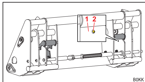
Abb. 85 Hochgeschwenkte Anlagen (Ansicht von hinten)
