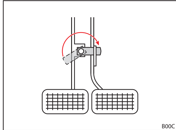
Abb. 42 Bremspedale koppeln
