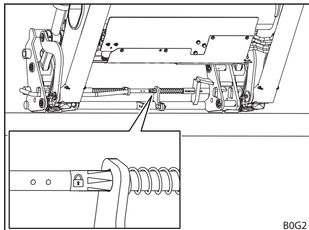
Abb. 77 Werkzeug-Verriegelung anhand des Aufklebers prüfen (Kombi-Wechselrahmen Euro-FR)
