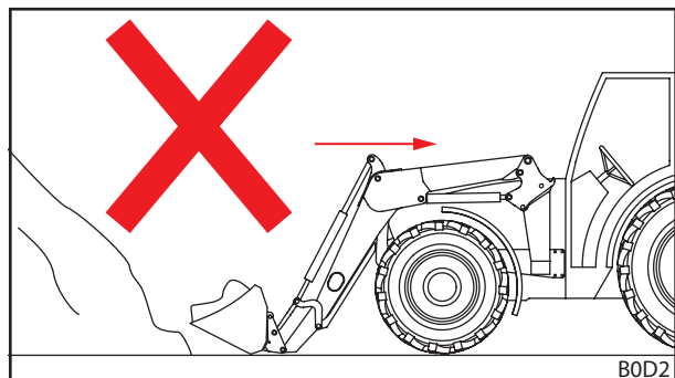
Abb. 106 Rückwärtsfahren unter Last – falsch
