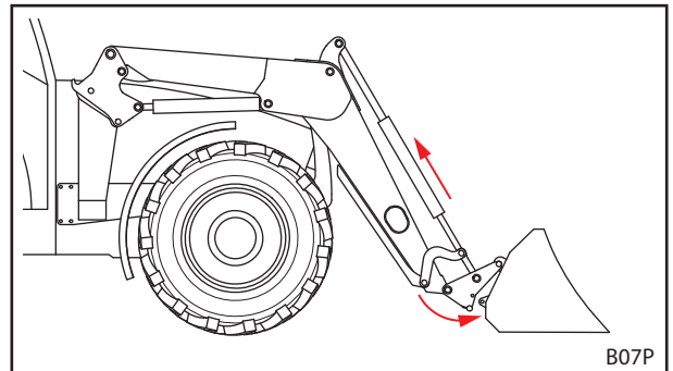
Abb. 91 Einhaken
