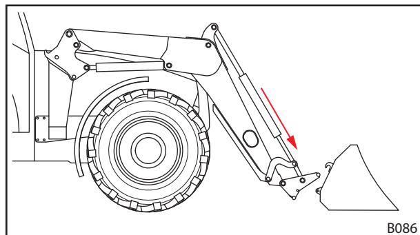
Abb. 89 Schwinde positionieren
