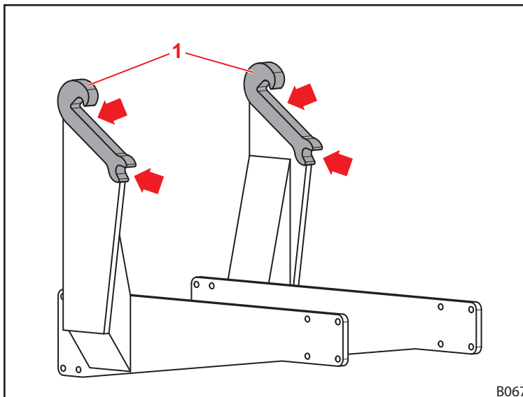
Abb. 108 Schmierstellen Frontlader-Aufnahmen
