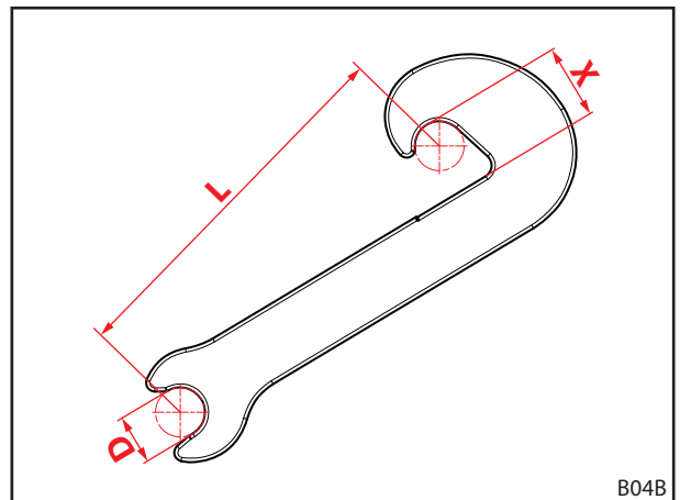
Abb. 111 Verschleißmaße des Fanghakens
