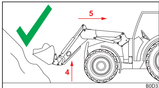
Abb. 107 Rückwärtsfahren unter Last – richtig
