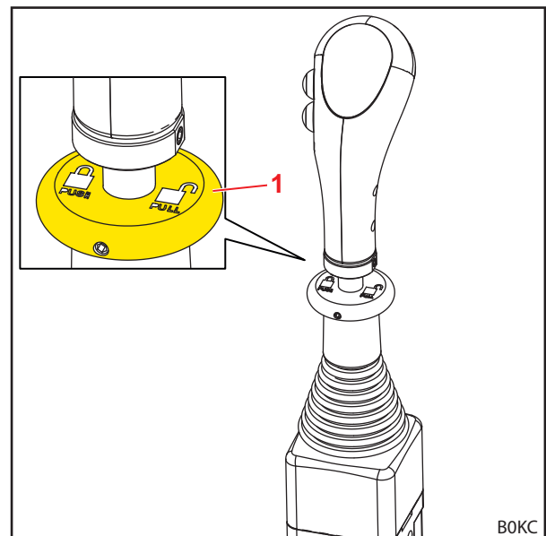
Abb. 61 Verriegelung des Bedienhebels (vertikale Verriegelung)
