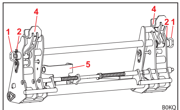
Abb. 19 Kombi-Wechselrahmen Euro-FR (vorbereitet für FR-Werkzeug)
