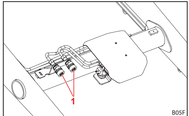
Abb. 38 Zusätzlicher 3. Steuerkreis
