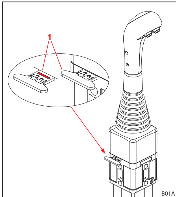
Abb. 60 Verriegelung des Bedienhebels (horizontale Verriegelung)
