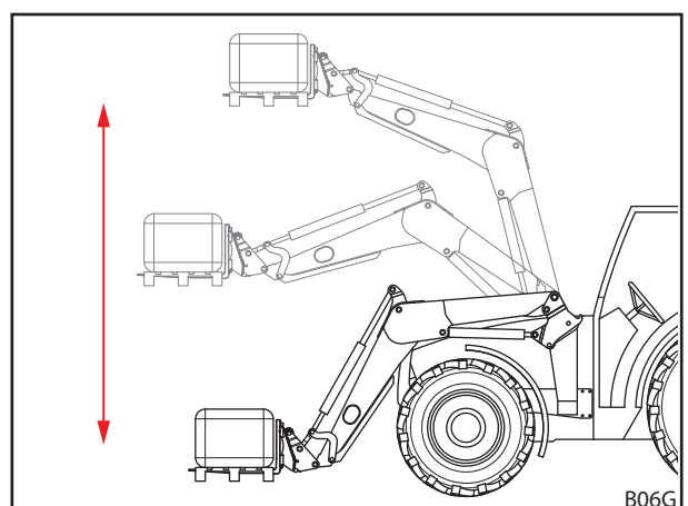
Abb. 32 Mechanische Parallelführung
