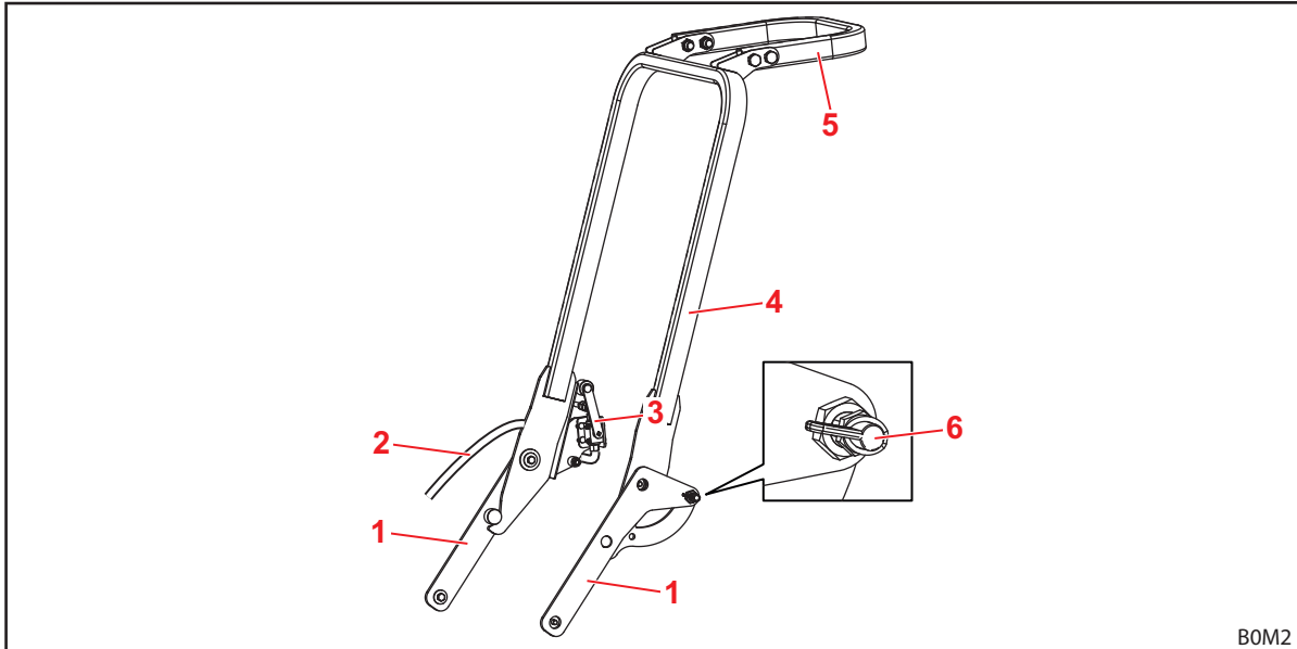
Abb. 11 Operator Protective Guard, OPG (beispielhafte Abbildung)
