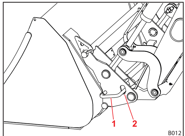
Abb. 75 Mechanische Werkzeug-Verriegelung
