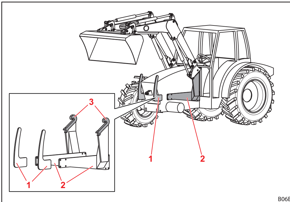
Abb. 12 Anbausatz für Traktor
