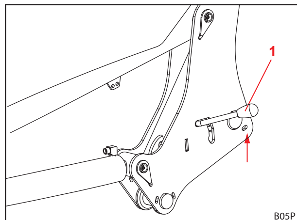
Abb. 53 Frontlader-Verriegelung öffnen
