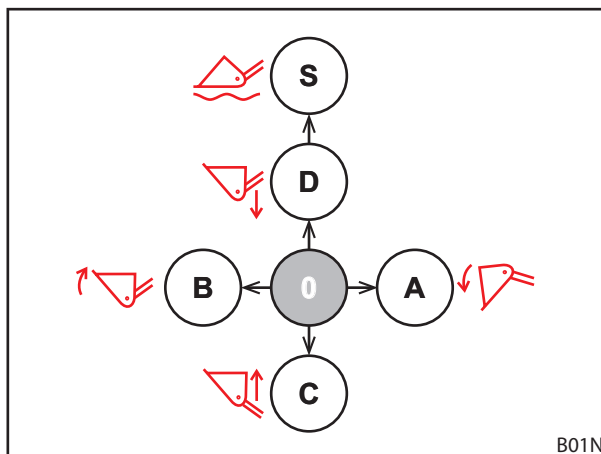
Abb. 57 Belegung bei einem Bedienhebel
