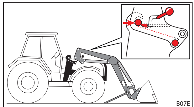
Abb. 47 Traktor in Schwinge einfahren
