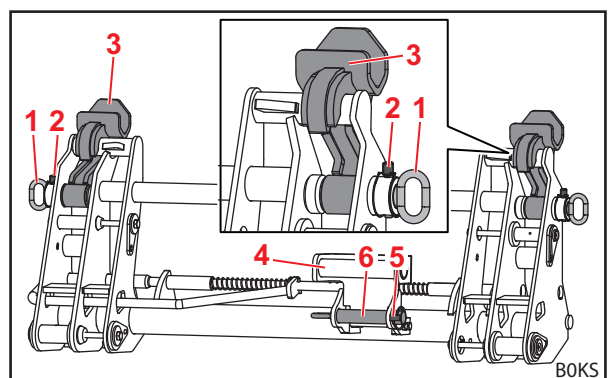
Abb. 87 Adapter in Arbeitsposition (Wechselrahmen vorbereitet für FR-Werkzeug)
