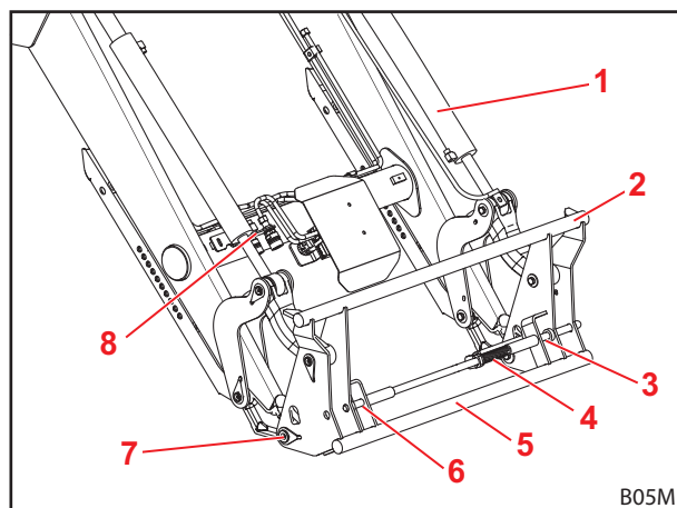
Abb. 13 Euro-Wechselrahmen
