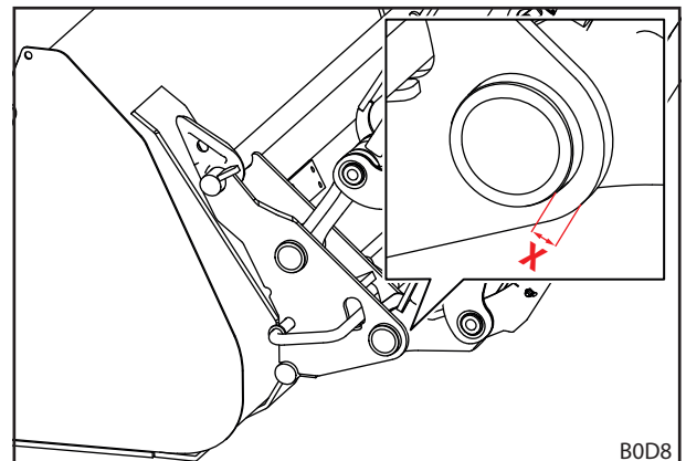
Abb. 113 Verschleißmaß des Wechselrahmens
