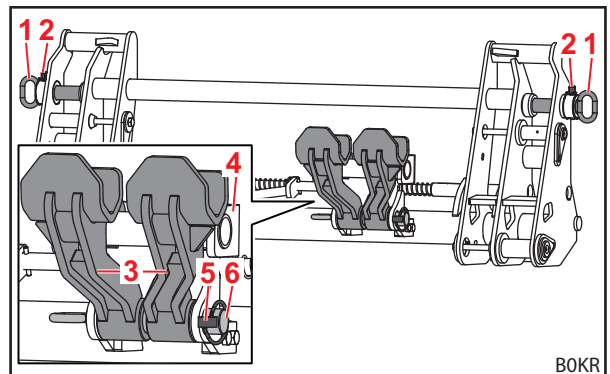
Abb. 86 Adapter in Parkposition (Wechselrahmen vorbereitet für Euro-Werkzeug)
