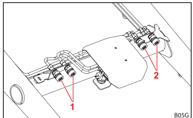
Abb. 39 Zusätzlicher 4. Steuerkreis
