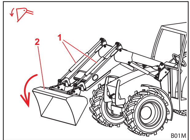
Abb. 29 Schütten-Funktion
