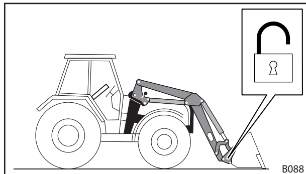
Abb. 94 Werkzeug-Verriegelung öffnen
