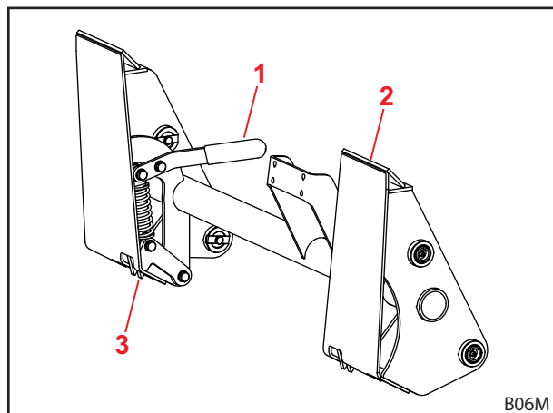
Abb. 25 Mechanische Werkzeug-Verriegelung an Skid-Steer-Wechselrahmen
