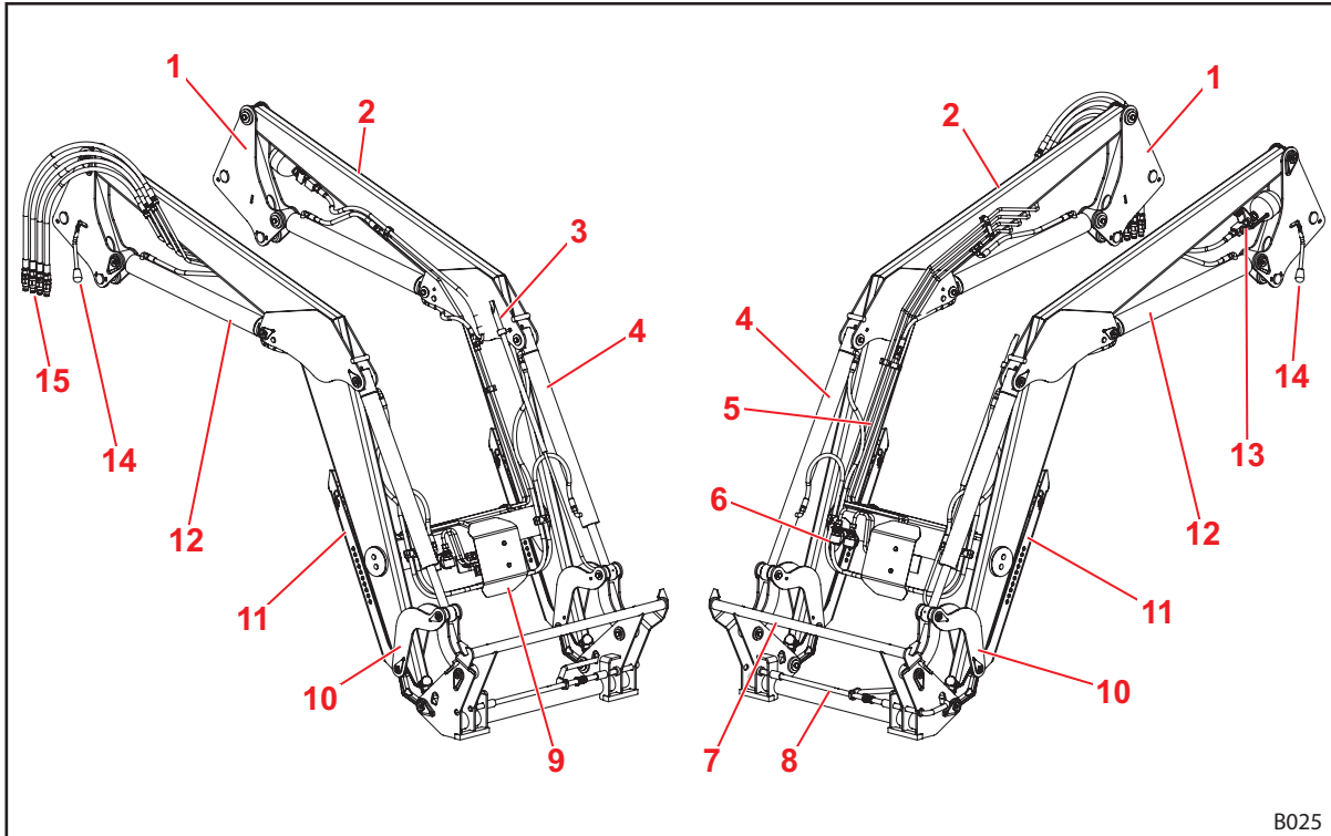
Abb. 9 Frontlader H (ohne mechanische Parallelführung)
