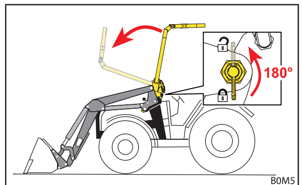
Abb. 34 OPG herunterklappen
