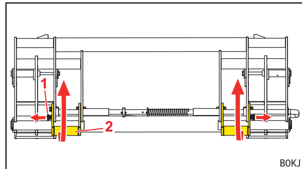
Abb. 84 Anlagen hochschwenken
