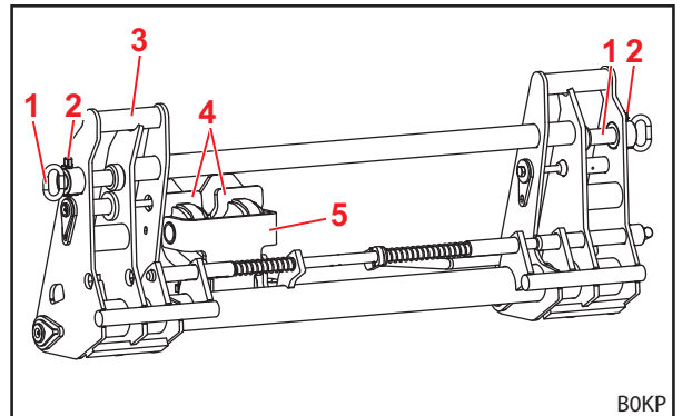
Abb. 18 Kombi-Wechselrahmen Euro-FR (vorbereitet für Euro-Werkzeug)
