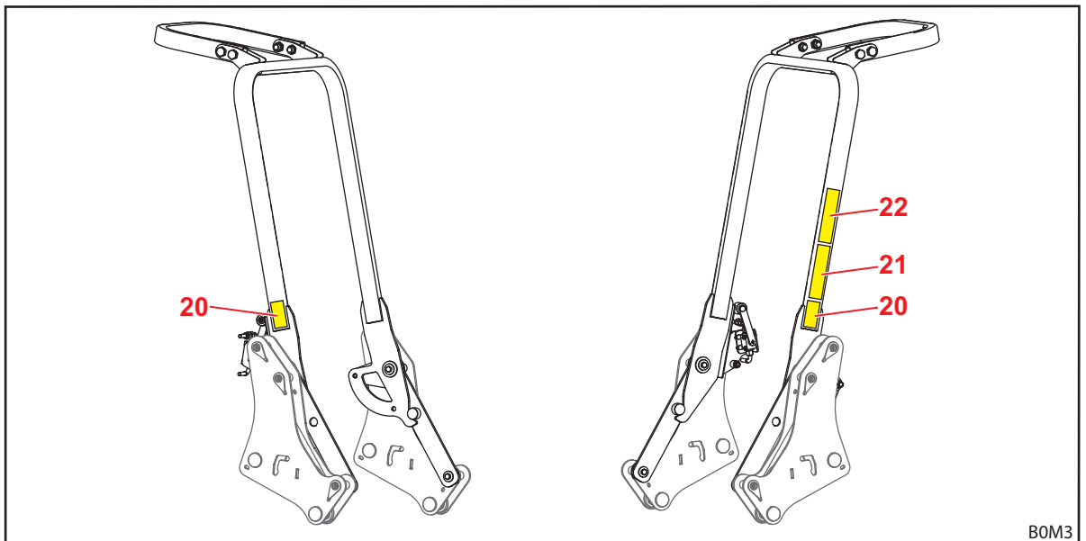
Abb. 7 OPG für Traktoren mit hinten angebrachter 2-Pfosten-Umsturzschutzvorrichtung (beispielhafte Abbildung)
