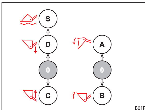
Abb. 58 Belegung bei zwei Bedienhebeln
