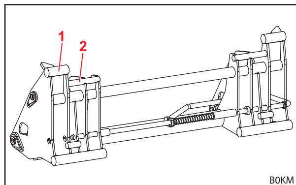
Abb. 17 Kombi-Wechselrahmen Euro-Alö3
