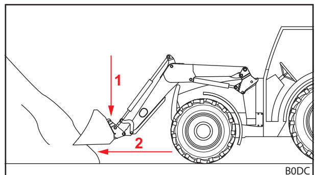
Abb. 104 Frontlader absenken und gerade in Ladegut einfahren
