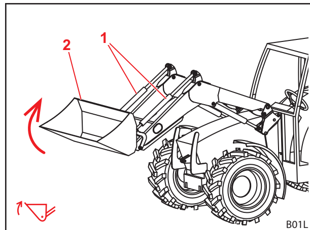
Abb. 28 Schöpfen-Funktion
