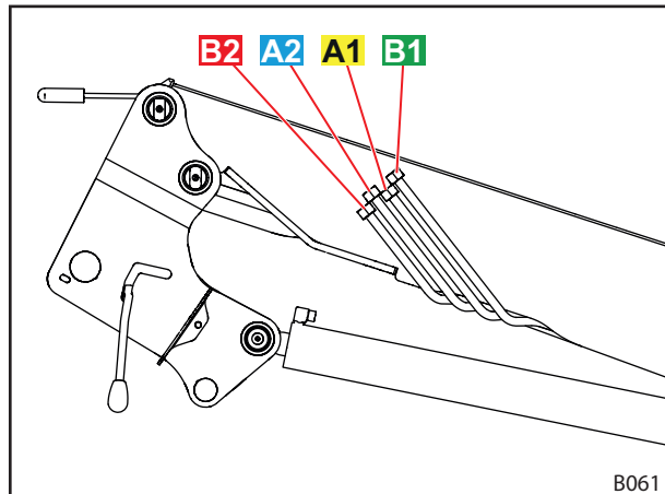
Abb. 20 Hydraulikleitungen
