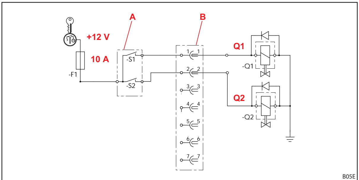
Abb. 121 Elektro-Schaltbild
