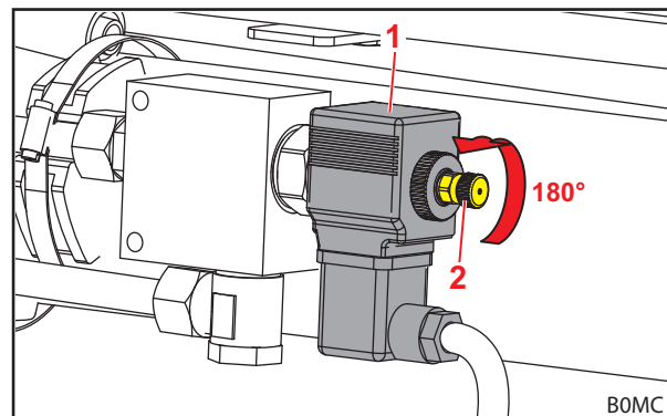
Abb. 33 Ventil öffnen
