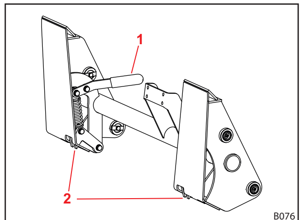
Abb. 80 Werkzeug-Verriegelung am Skid-Steer-Wechselrahmen
