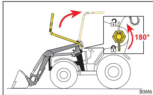
Abb. 36 OPG hochklappen
