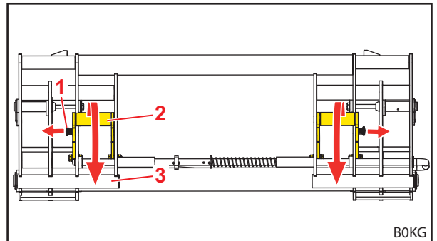
Abb. 82 Anlagen herunterschwenken
