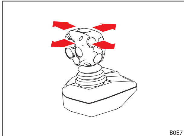
Abb. 68 Joystick in alle Endlagen bewegen
