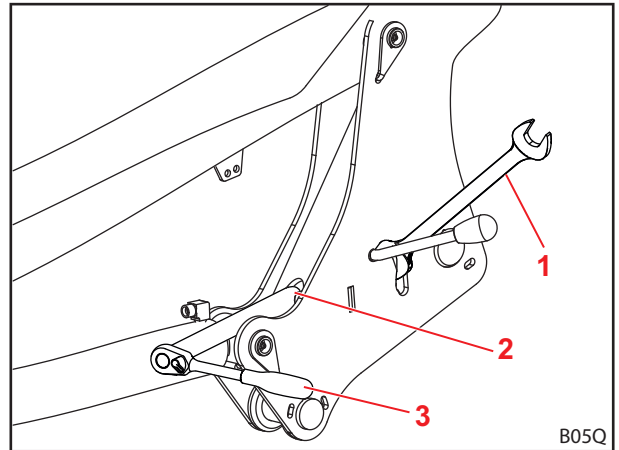
Abb. 54 Werkzeug anlegen
