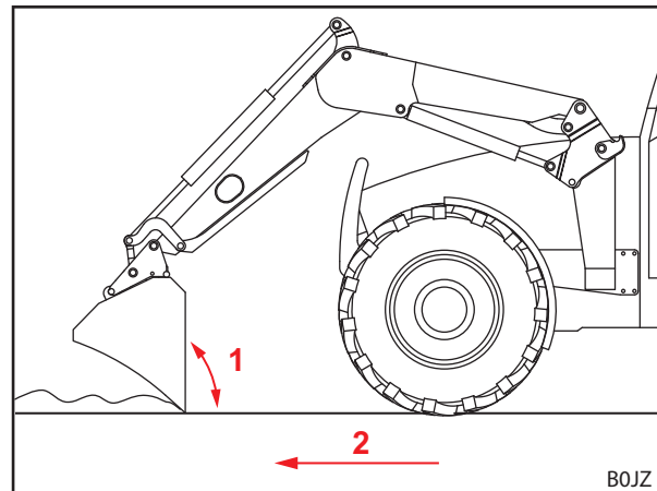
Abb. 103 Räumen
