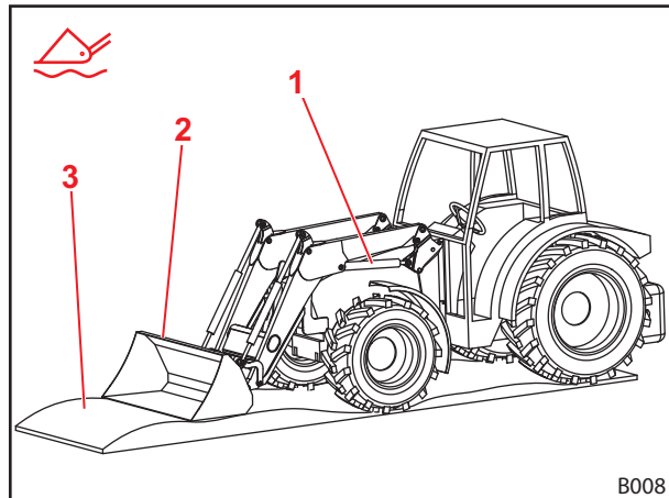
Abb. 30 Frontlader in Schwimmstellung
