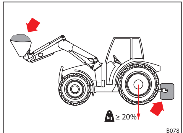
Abb. 43 Belastung bei Frontladerarbeiten
