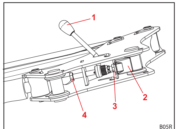
Abb. 56 Ansicht der Frontlader-Verriegelung von unten
