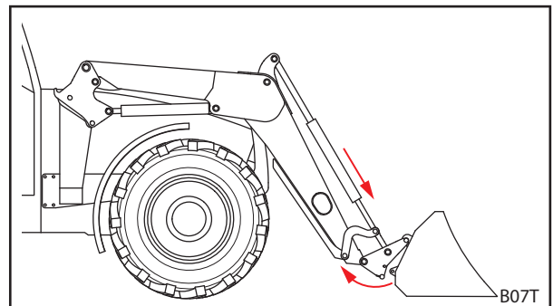
Abb. 100 Wechselrahmen aushaken
