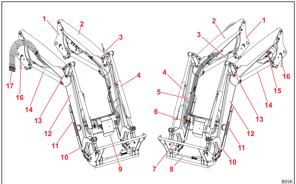
Abb. 10 Frontlader P (mit mechanischer Parallelführung)
