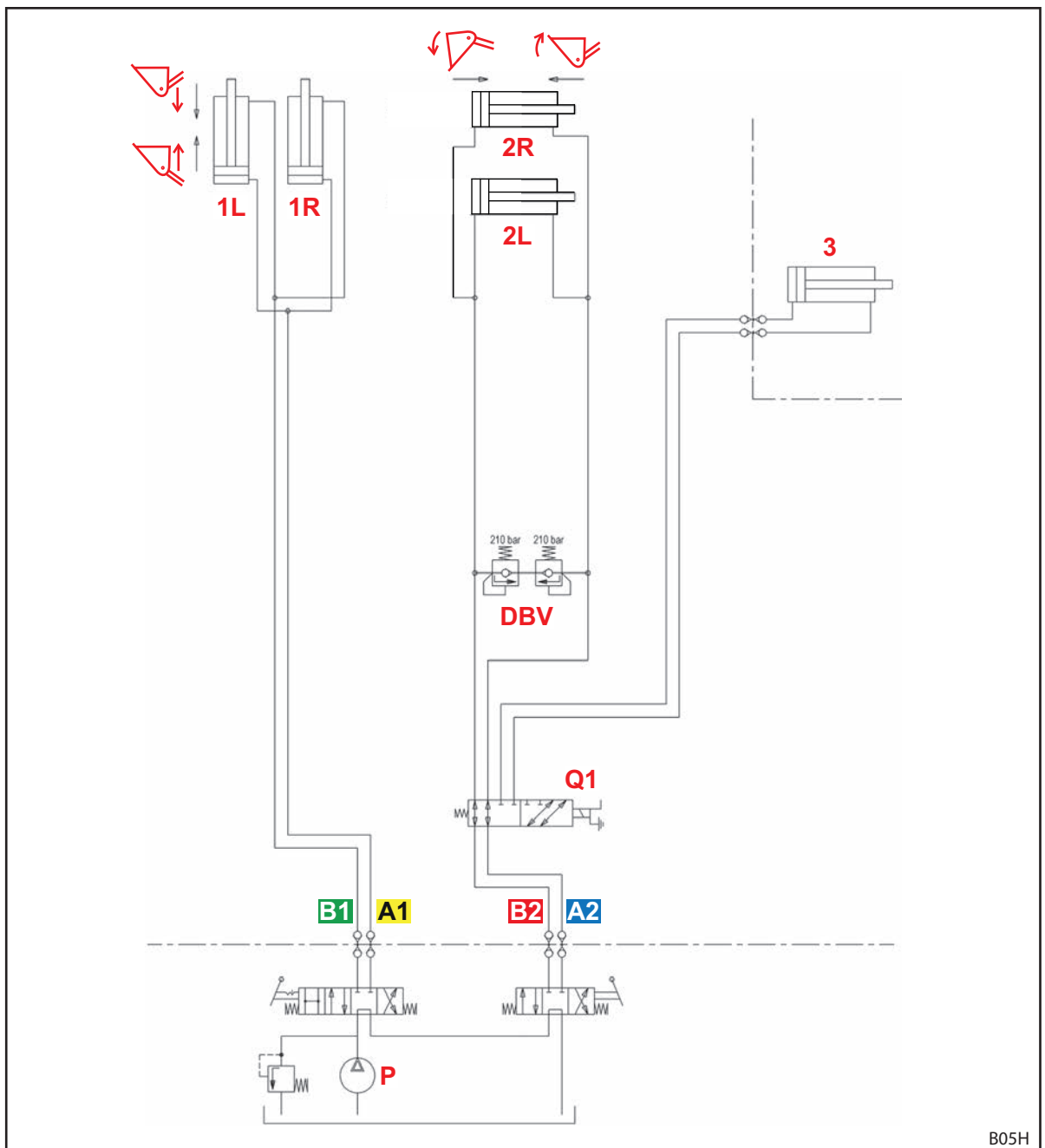
Abb. 119 Hydraulikplan H
