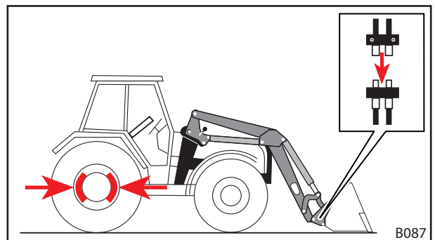
Abb. 93 Hydraulikleitungen des Werkzeuges mit Frontlader-Kupplungen verbinden
