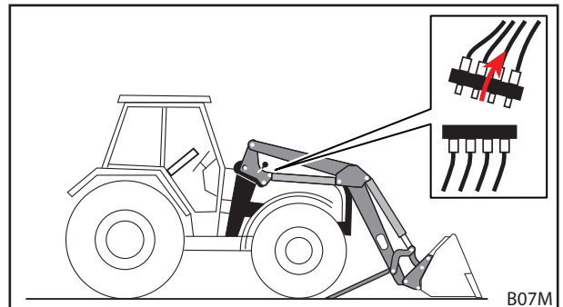
Abb. 117 Hydraulik abkoppeln
