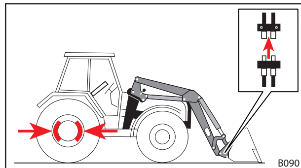
Abb. 99 Hydraulikleitungen lösen
