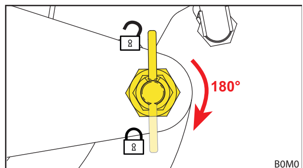
Abb. 35 Rastriegel in verriegelte Position bringen
