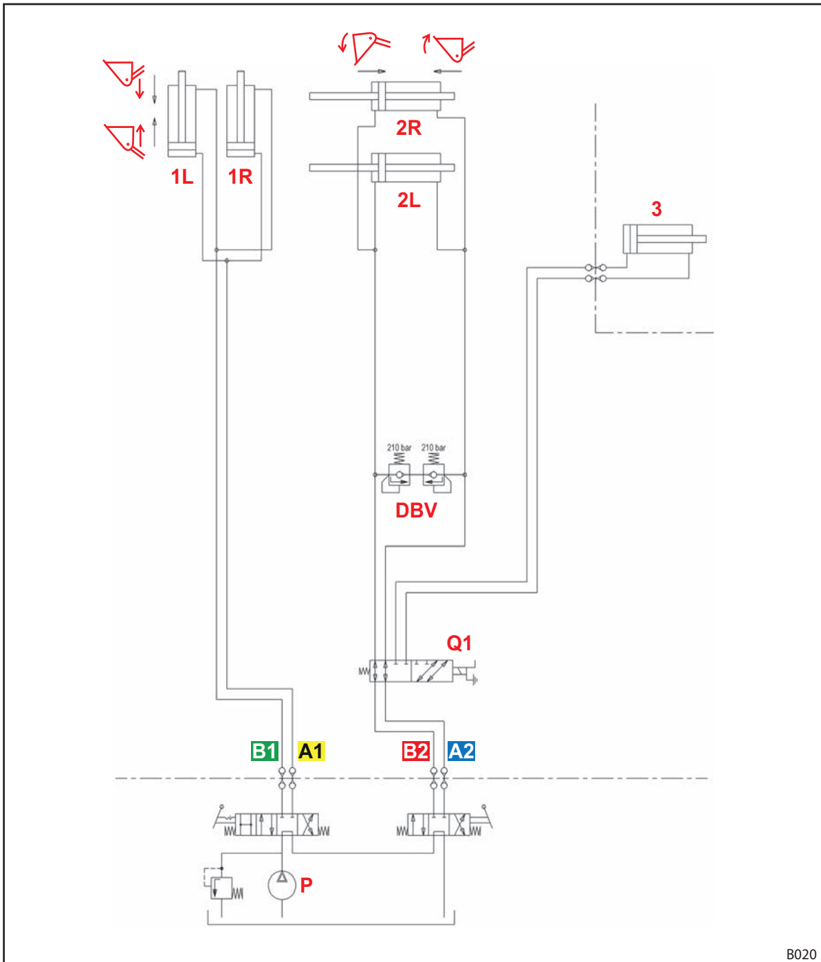
Abb. 120 Hydraulikplan P
