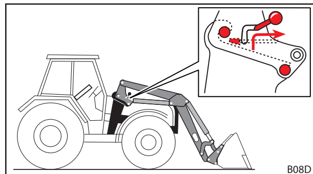
Abb. 115 Frontlader-Verriegelung lösen
