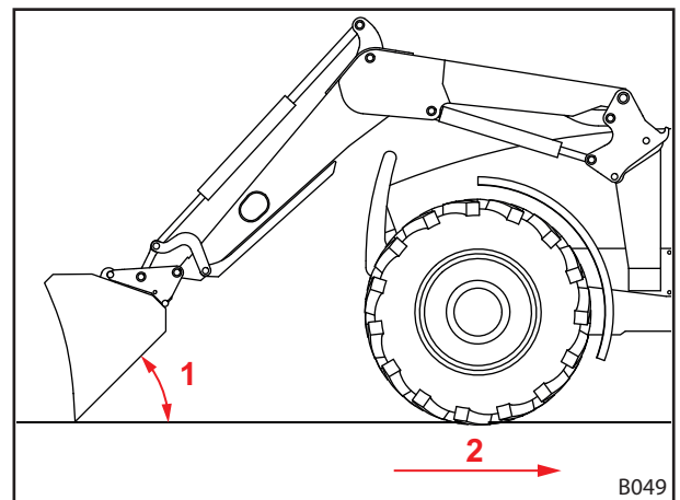
Abb. 102 Rückwärts planieren
