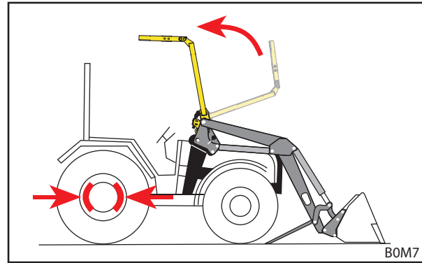
Abb. 49 OPG hochklappen
