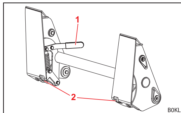
Abb. 14 Skid-Steer-Wechselrahmen
