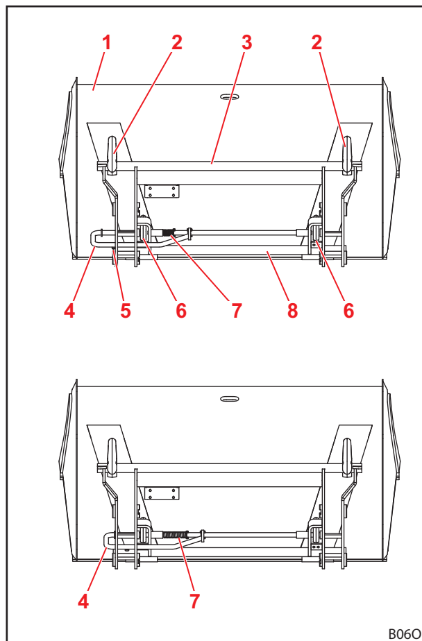
Abb. 24 Geöffnete (oben) und geschlossene (unten) Verriegelung
