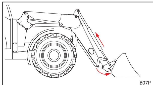
Abb. 96 Einhängen
