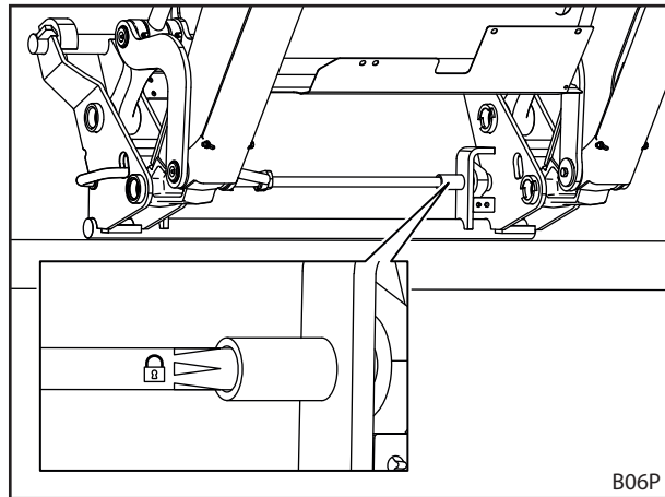
Abb. 76 Werkzeug-Verriegelung anhand des Aufklebers prüfen
