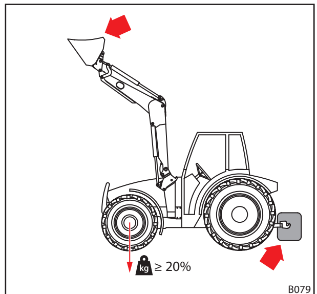
Abb. 44 Belastung bei Straßenfahrten
